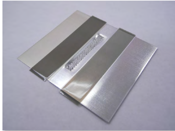
上：[アルミタブ t =0.4 mm] 下：[Niメッキ銅タブ t =0.2 mm]
