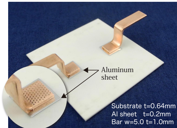
★ [アルミナ基板 & 銅ブスバー] アルミシートを挟んで接合
