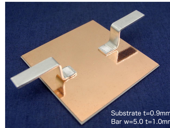
★ [AMC 基板 & アルミブスバー]
