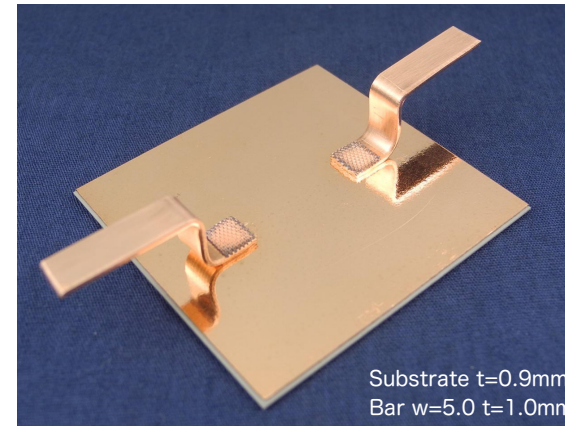
★ [AMC 基板 & 銅ブスバー]
