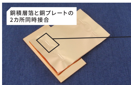
接合部拡大
