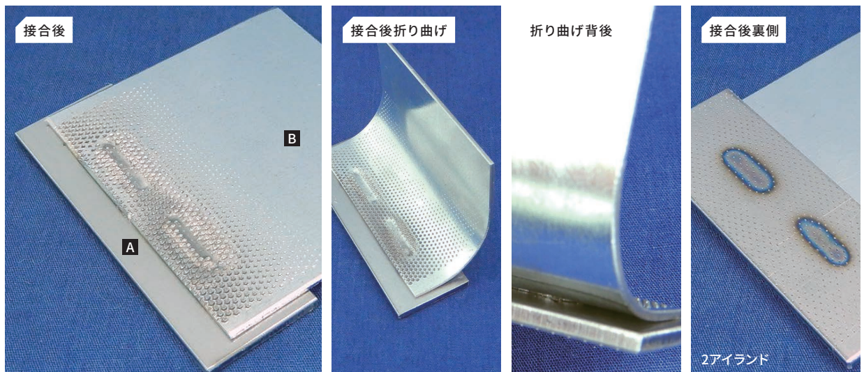
A ハイテン(t=2.3mm) B 亜鉛めっき鋼板(t=1.2mm)
