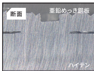
A ハイテン(t=2.3mm) B 亜鉛めっき鋼板(t=1.2mm)
