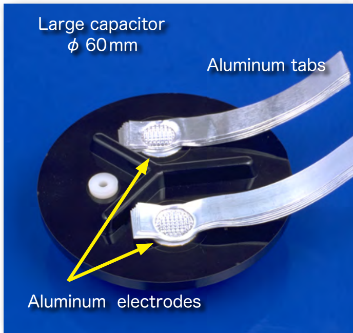
アルミタブと電極の直接接合
